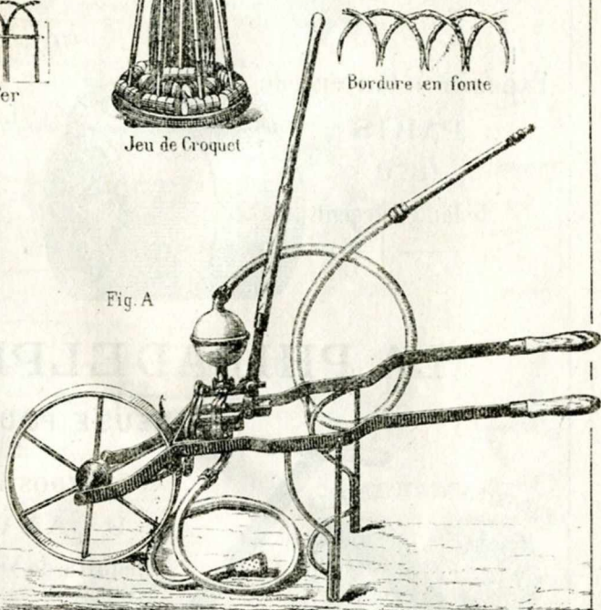
Pompe sur brouette aspirante et foulante
