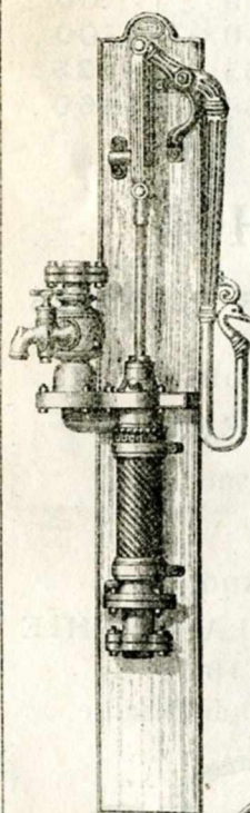
POMPE sur madrier aspirante et foulante
